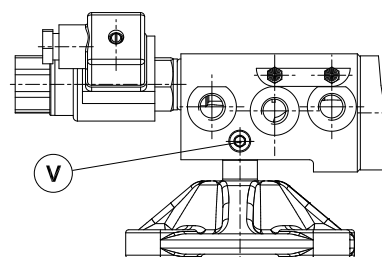
VUE DE DESSUS / TOPVIEW
