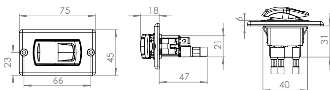
Interrupteur Comfort
